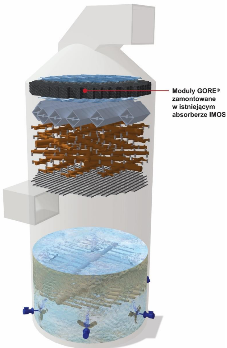
Instalacja w absorberze IMOS
